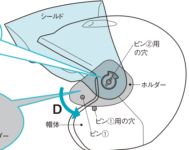
[図V] ホルダーを回転させピン①を差し込む
