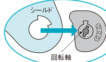
[図IV] ホルダーのピン②を差し込む
