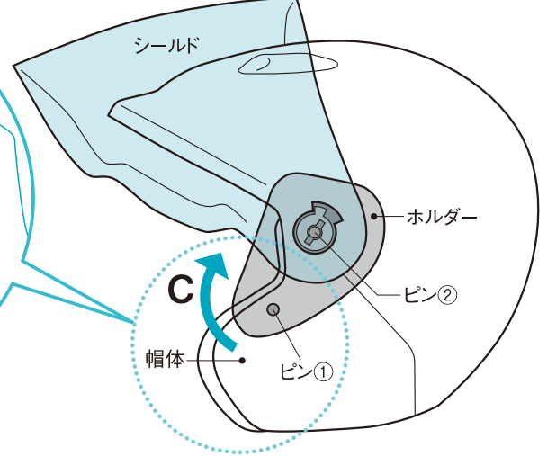
[図II] シールドの着脱の位置
