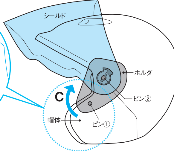
【図II】シールドの着脱の位置
