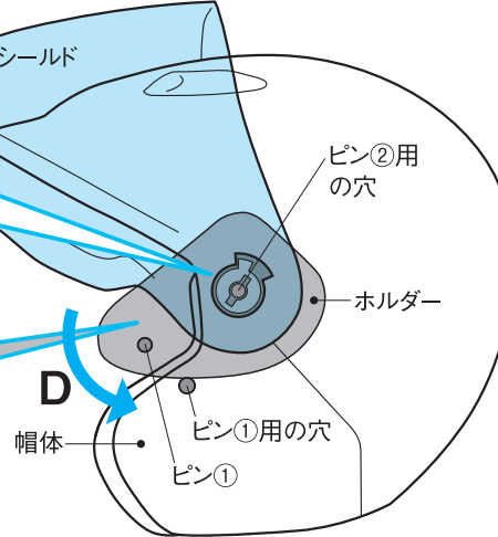
【図V】ホルダーを回転させピン①を差し込む
