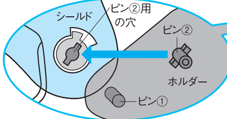
【図IV】ホルダーのピン②を差し込む
